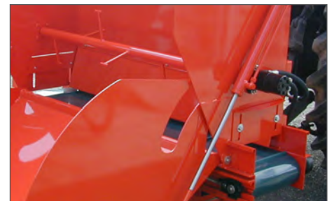
Hydraulisches Rührwerk und Mengenregulierung durch verstellbare Auswurfluken
